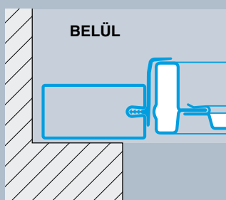
N80-as típus vasalat a nyílás mögött
