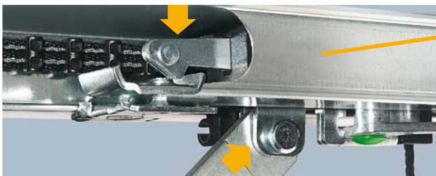
A kapu reteszelése a hajtósínben – Hörmann – szabadalom
