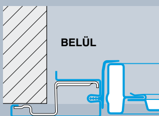
F80-as típus vasalat a nyílás mögött
