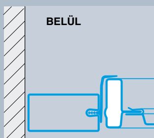
N80-as típus vasalat a nyílásban
